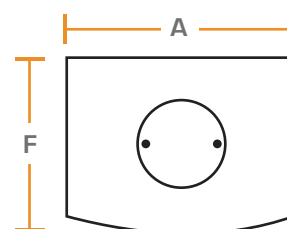
Boven aanzicht
