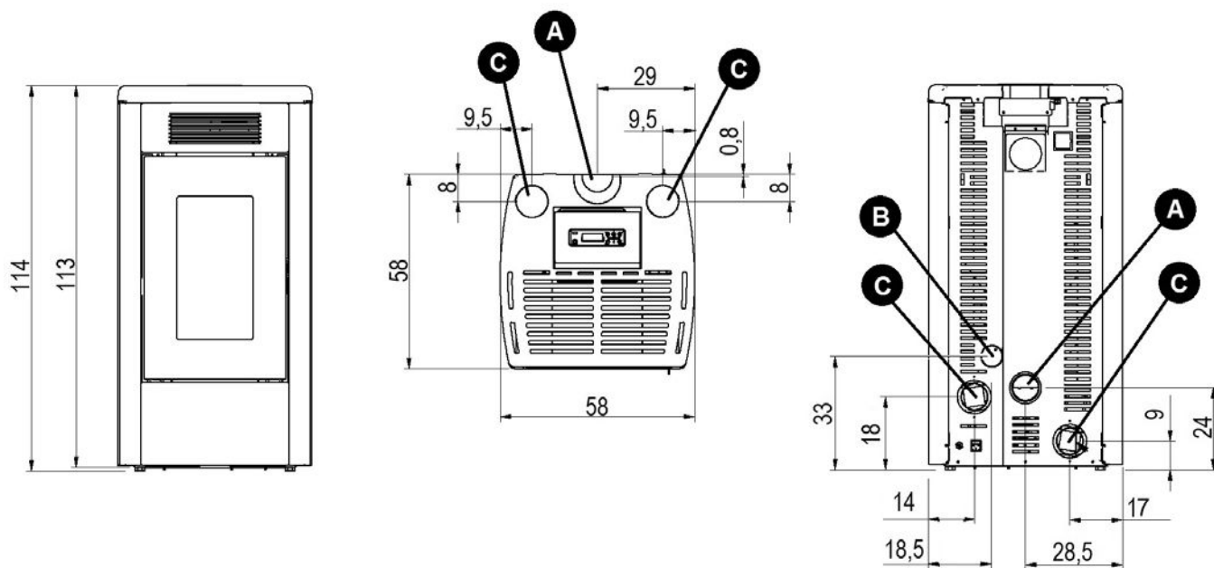
Fig. 12 - Algemene afmetingen: Atena³ Plus 12/14
