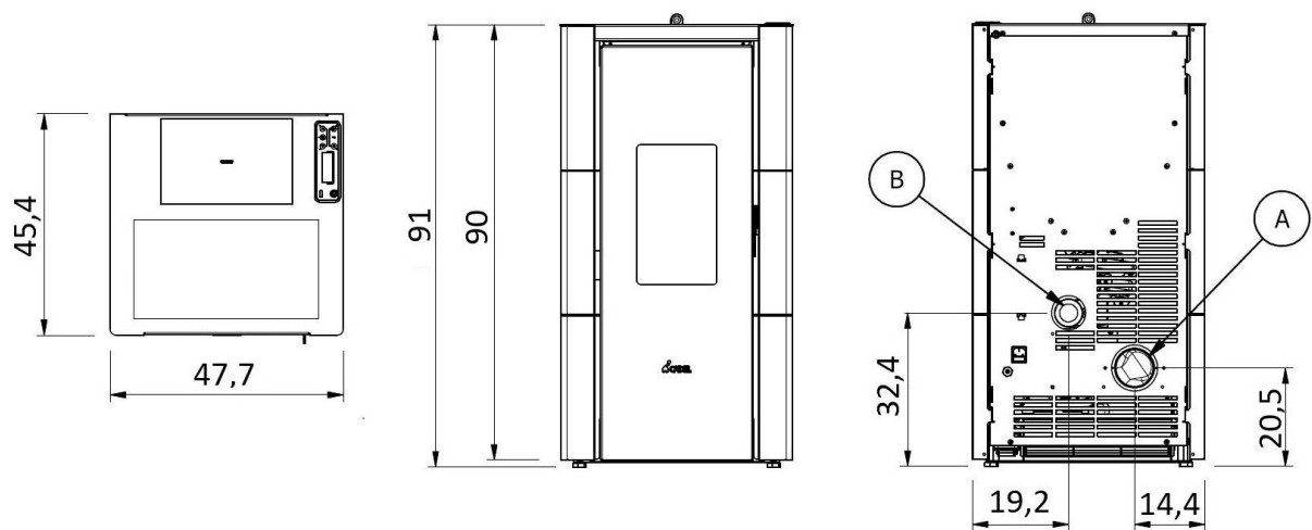
Fig. 15 - Algemene afmetingen: CRISTAL³ 7-7.0
