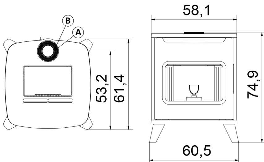
Fig. 13 - Algemene afmetingen: HUBLLOT 6 UP
