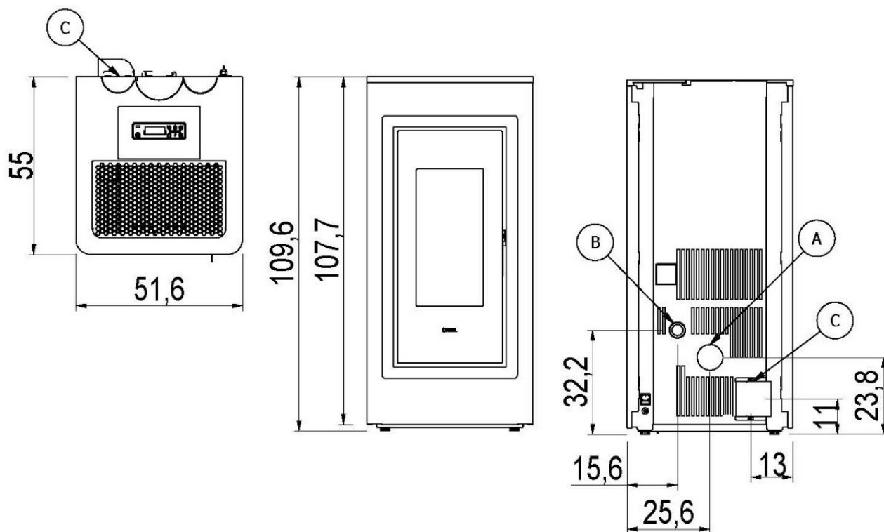
Fig. 13 - Algemene afmetingen: Kobe 11 - Kobe Plus 11
