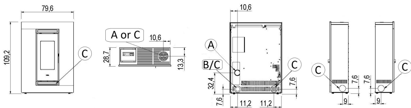
Fig. 13 - Algemene afmetingen: Luce Plus 9
