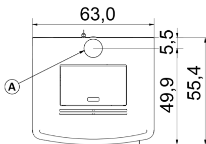
Fig. 12 - Algemene afmetingen: MAGRITTE 6
