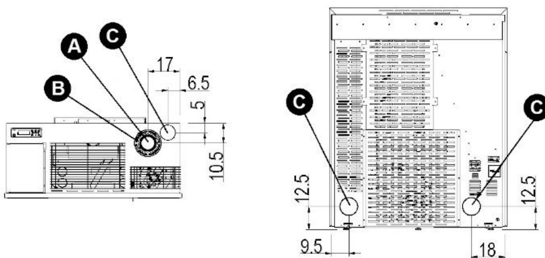
Fig. 16 - Algemene afmetingen: Mithos3 Plus 12/14
