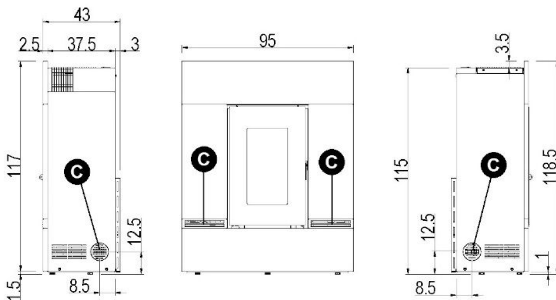
Fig. 15 - Algemene afmetingen: Mithos³ Plus 12/14
