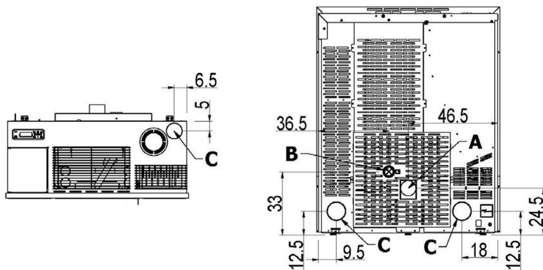
Fig. 18 - Algemene afmetingen: Mithos Plus 12/14 PS
