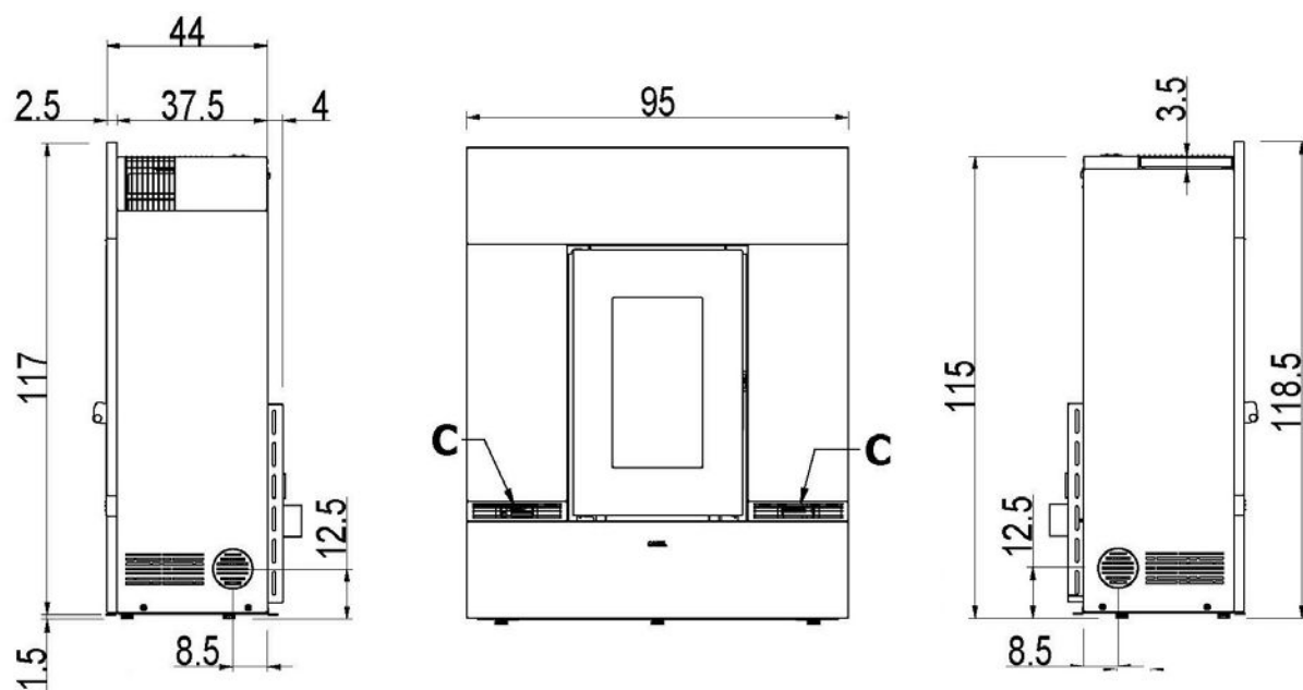
Fig. 17 - Algemene afmetingen: Mithos Plus 12/14 PS
