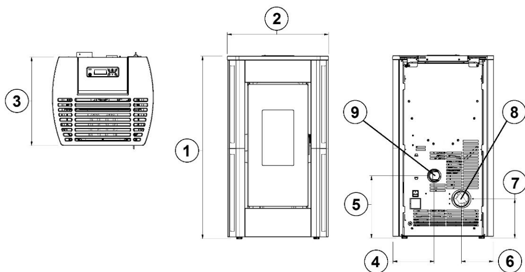
Fig. 14 - Algemene afmetingen: PERLA³ 7 - 7.0
