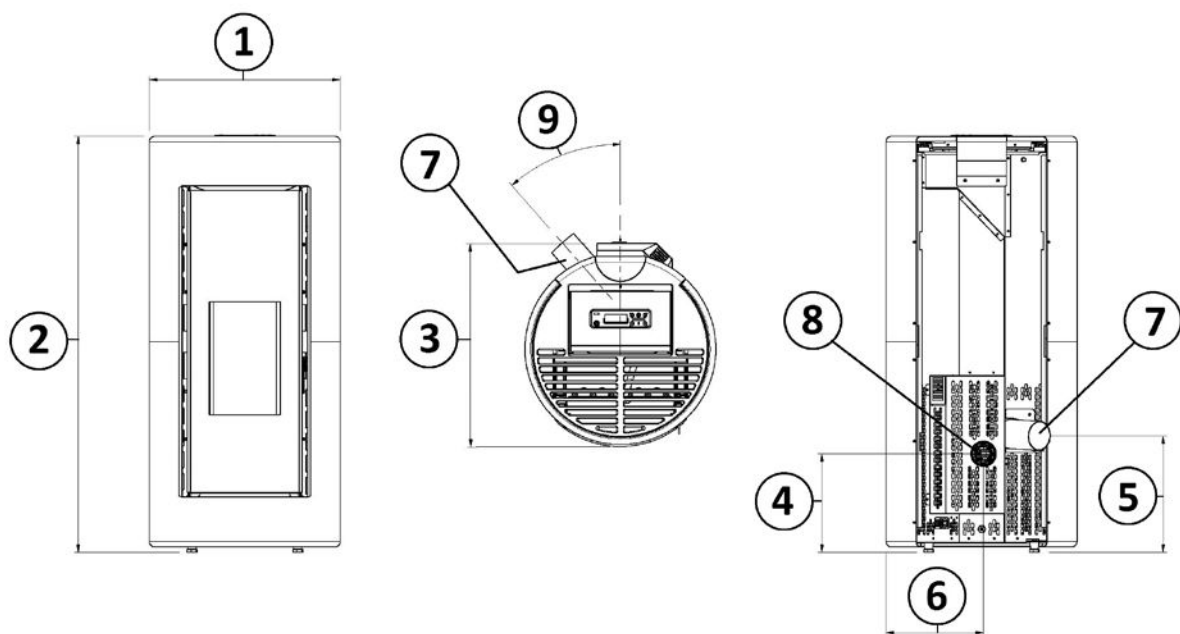
Fig. 16 - Algemene afmetingen: Shell ® Ps
