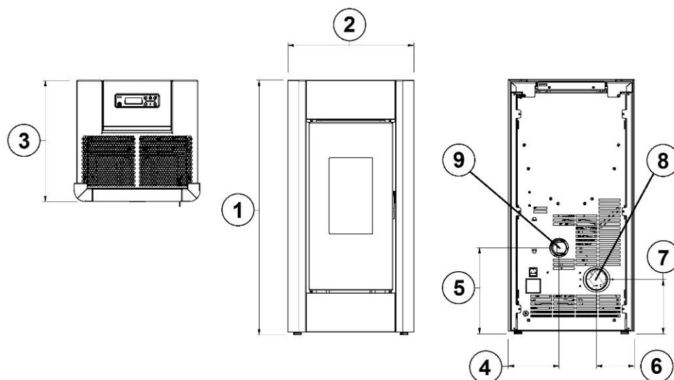
Fig. 13 - Algemene afmetingen: SWEET³ 7-7.0
