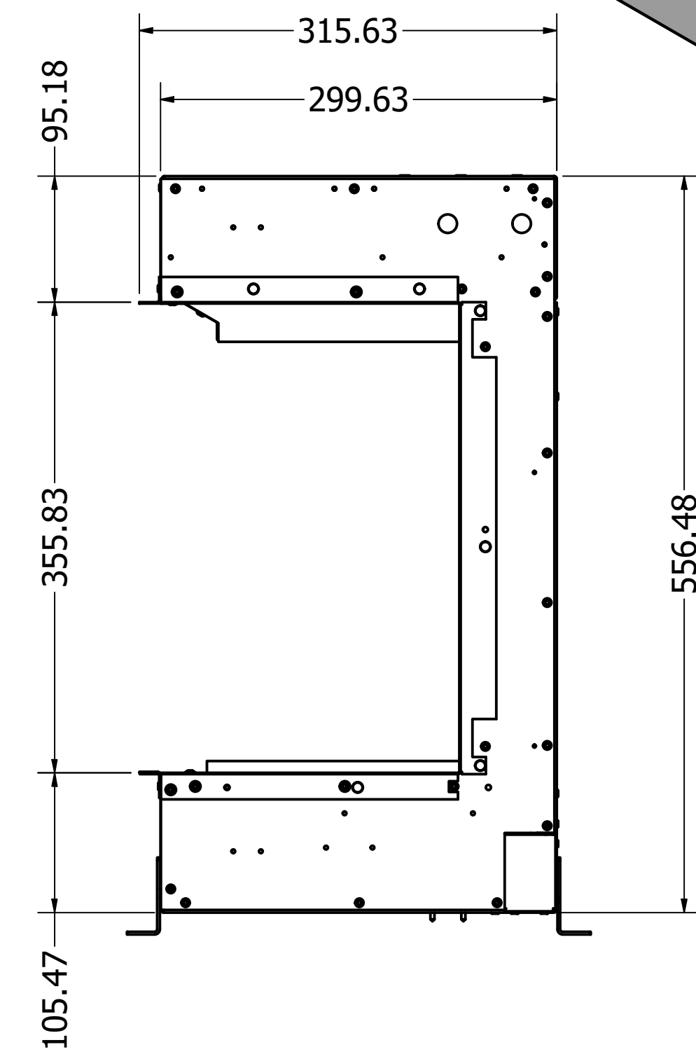
Club 125e 3 sided Alle maten in mm All sizes in mm Alle Größen in mm
