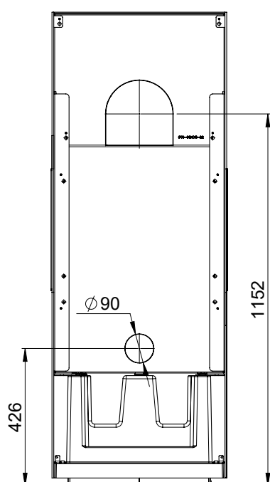
Nordpeis Box Base N-20U = Air
