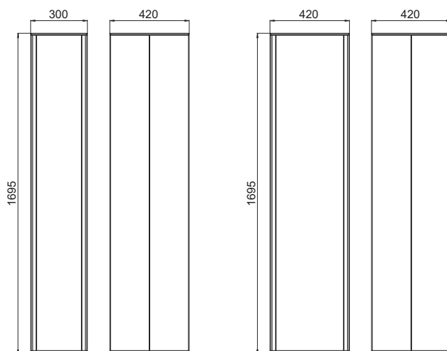
Vooraanzicht Zijaanzicht
