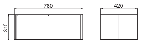
Vooraanzicht
