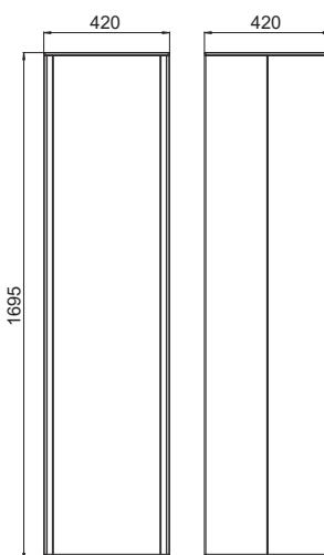
Vooraanzicht Zijaanzicht
