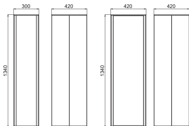
Vooraanzicht Zijaanzicht
