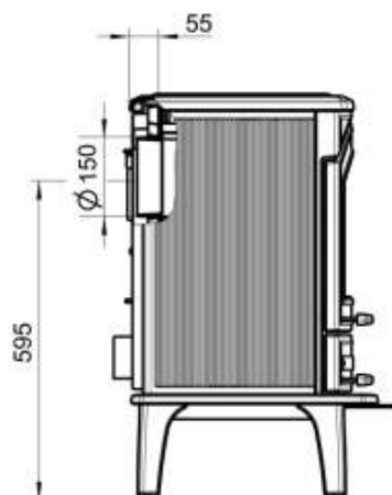
Achteraansluiting
